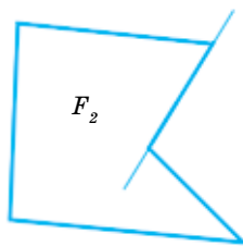
Невыпуклый многоугольник
